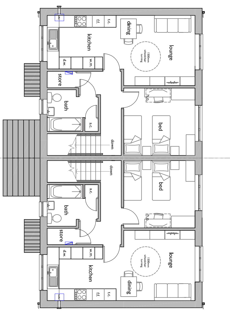
Cynllun Llwr Cynnal Arfaethedig 1:50 Proposed First Floor Plan 1:50
